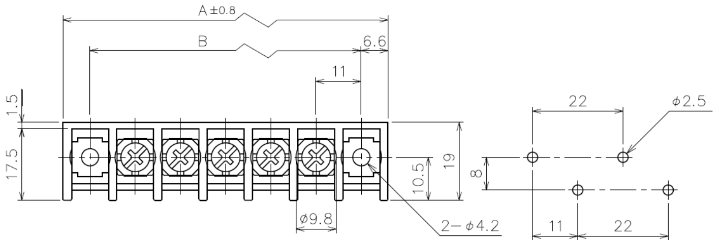
△ 基板取付穴寸法
